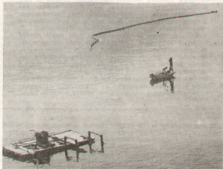
Постављање цијеви на морско дно
